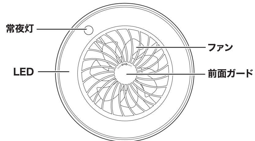
本体表面
